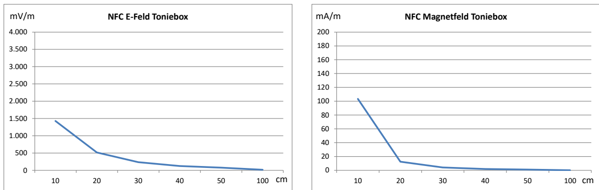
Abb. 4: Elektrische (links) und magnetische (rechts) Feldstärke des NFC-Signals als Funktion des Abstandes von der Toniebox (gemessen mit Spektrumanalysator und Peak-Detector, Spitzenwert)
