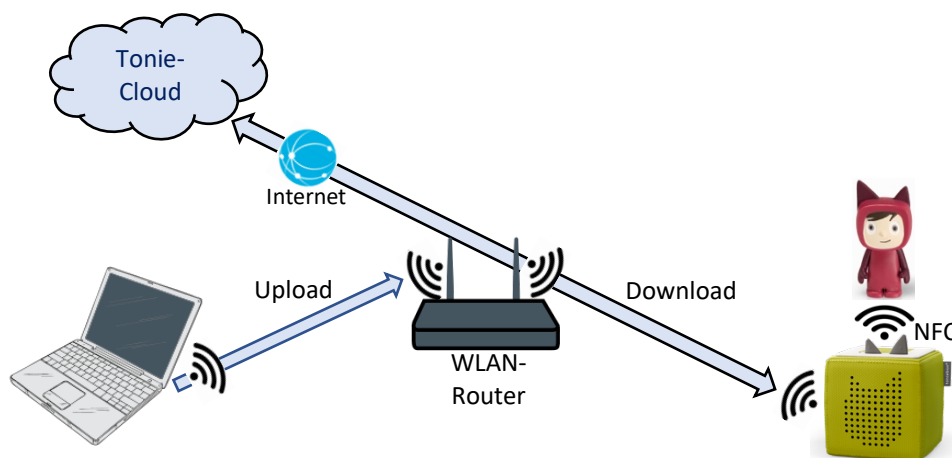
Abb. 2c: Funktionsprinzip der Toniebox mit Kreativ-Tonie, Upload in und Download aus der Tonie-Cloud per Internet, WLAN-Router und NFC
